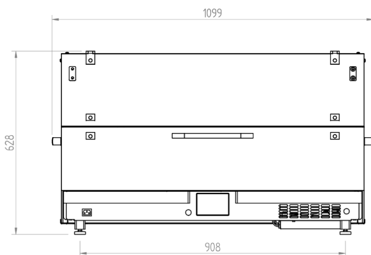
ALZADO
